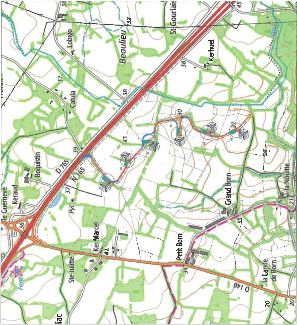
Figure 8 : Plan de masse général du projet de renouvellement sur fond IGN - Scénario avec les Vestas V110
